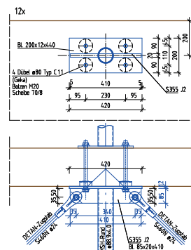
Anschluss Kippsteife mit Verband Achse B-D/2,3,6,7
