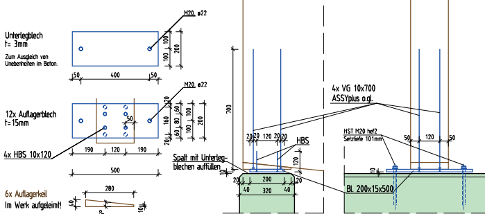
Auflager Binder Achse A / 2-7 Auflager Binder Achse E / 2-7
