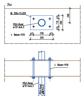
Anschluss Kippsteife Achse B-D/2-7
